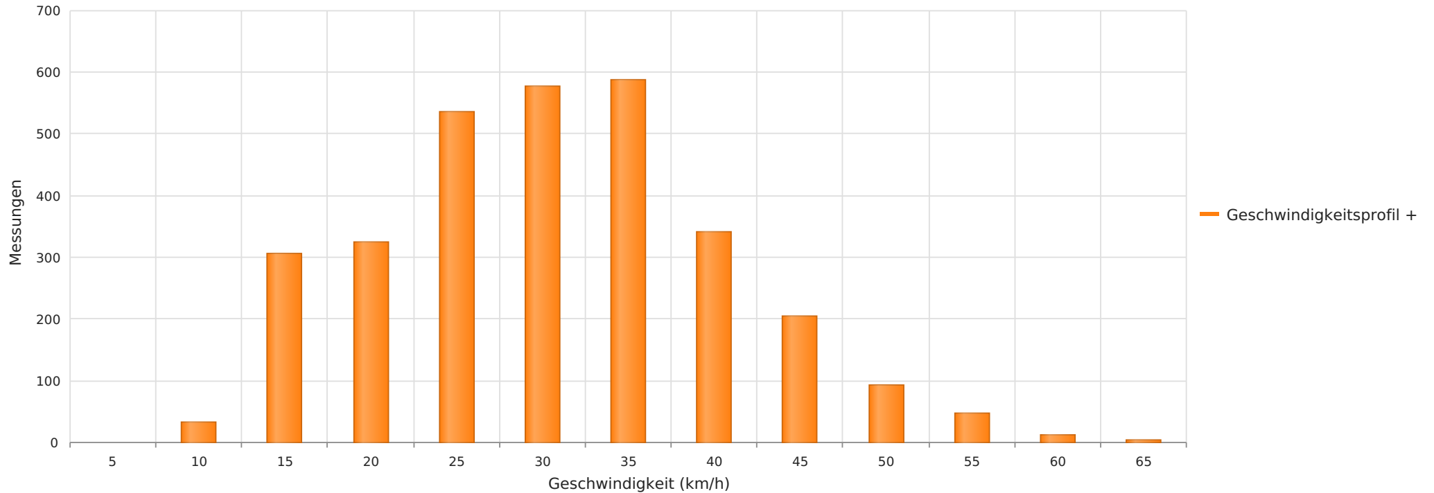
Hinterm Teich, Levern, Fahrtrichtung Osten, 30 km/h Beschränkung Anzahl der Messwerte vs. Geschwindigkeit
